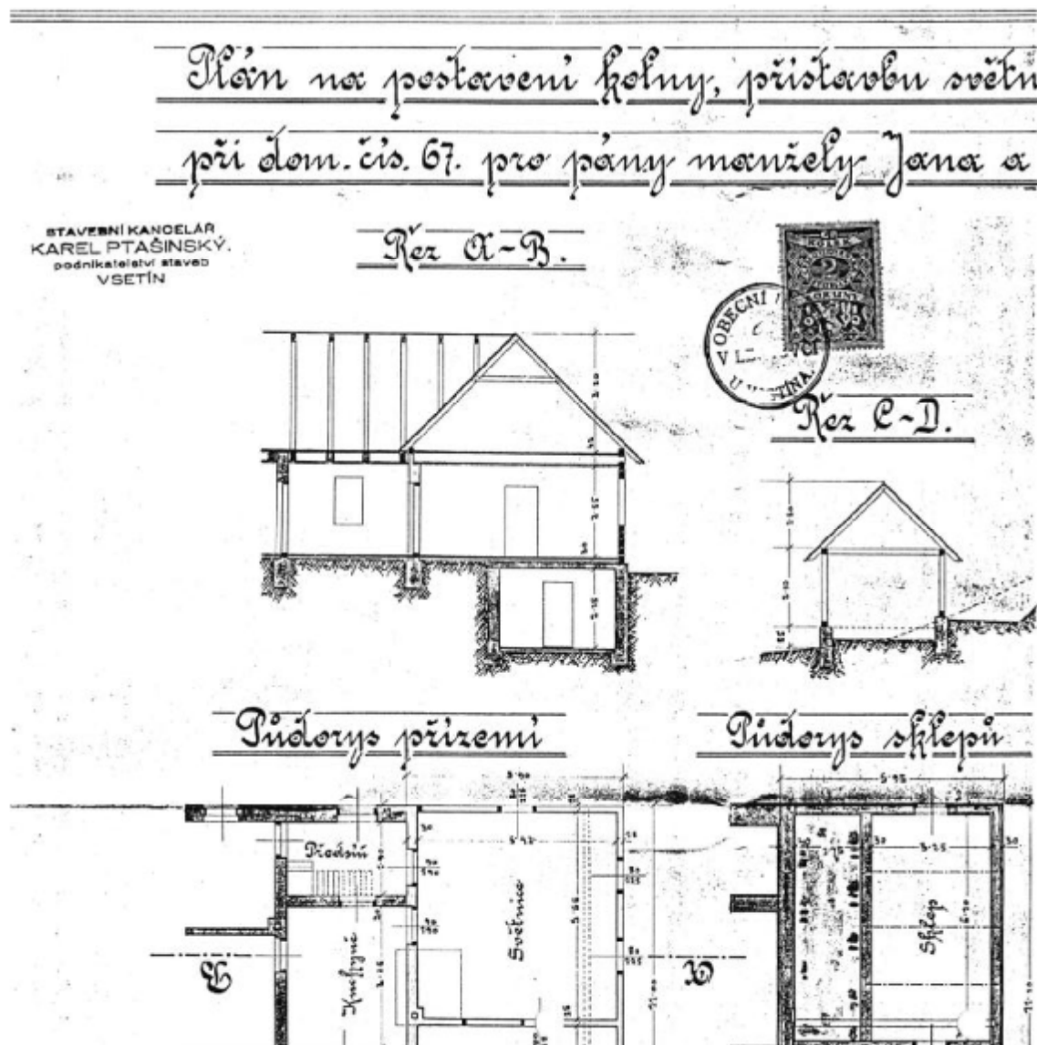
Plán na přístavbu domu Juříčkových z roku 1936, originál Obec Leskovec.
